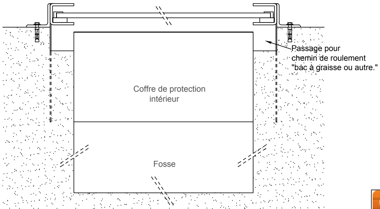
Coupe sur la largeur cas de figure principal
